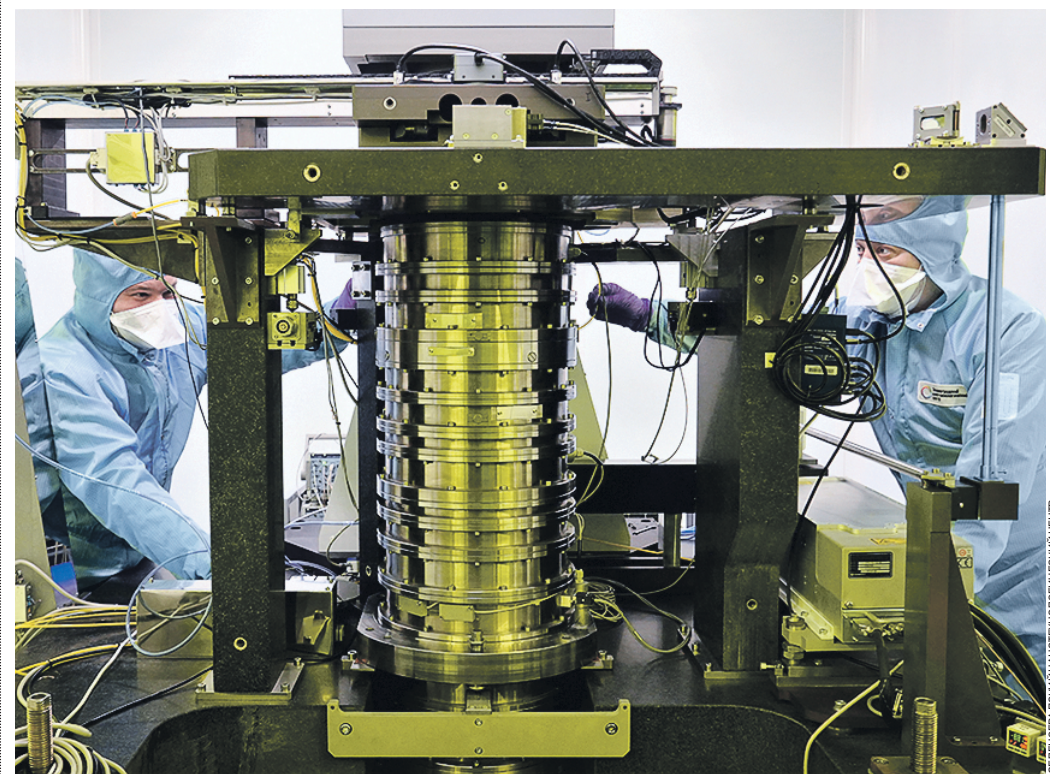
24 марта. Сотрудники Зеленоградского нанотехнологического центра представляют первый отечественный фотолитограф для изготовления чипов размером 350 нанометров
